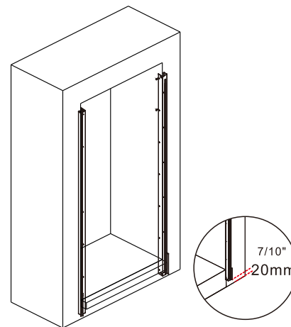
3 Fix the left outer frame bracket and the right outer frame bracket Fixez le support de cadre extérieur gauche et le support de cadre extérieur droit
